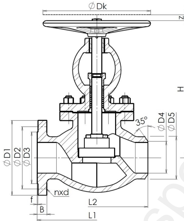
Main and connection dimensions / главные и присоед. Размеры
